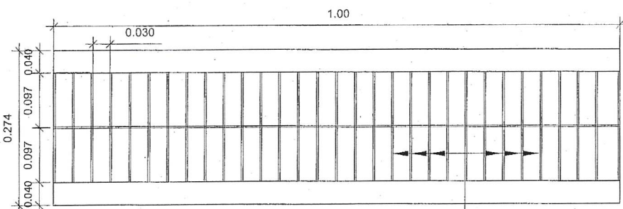
แปลนขยายฝาตะแกรงเหล็ก
