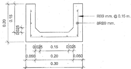
แบบขยายรางกีดเดอร์
