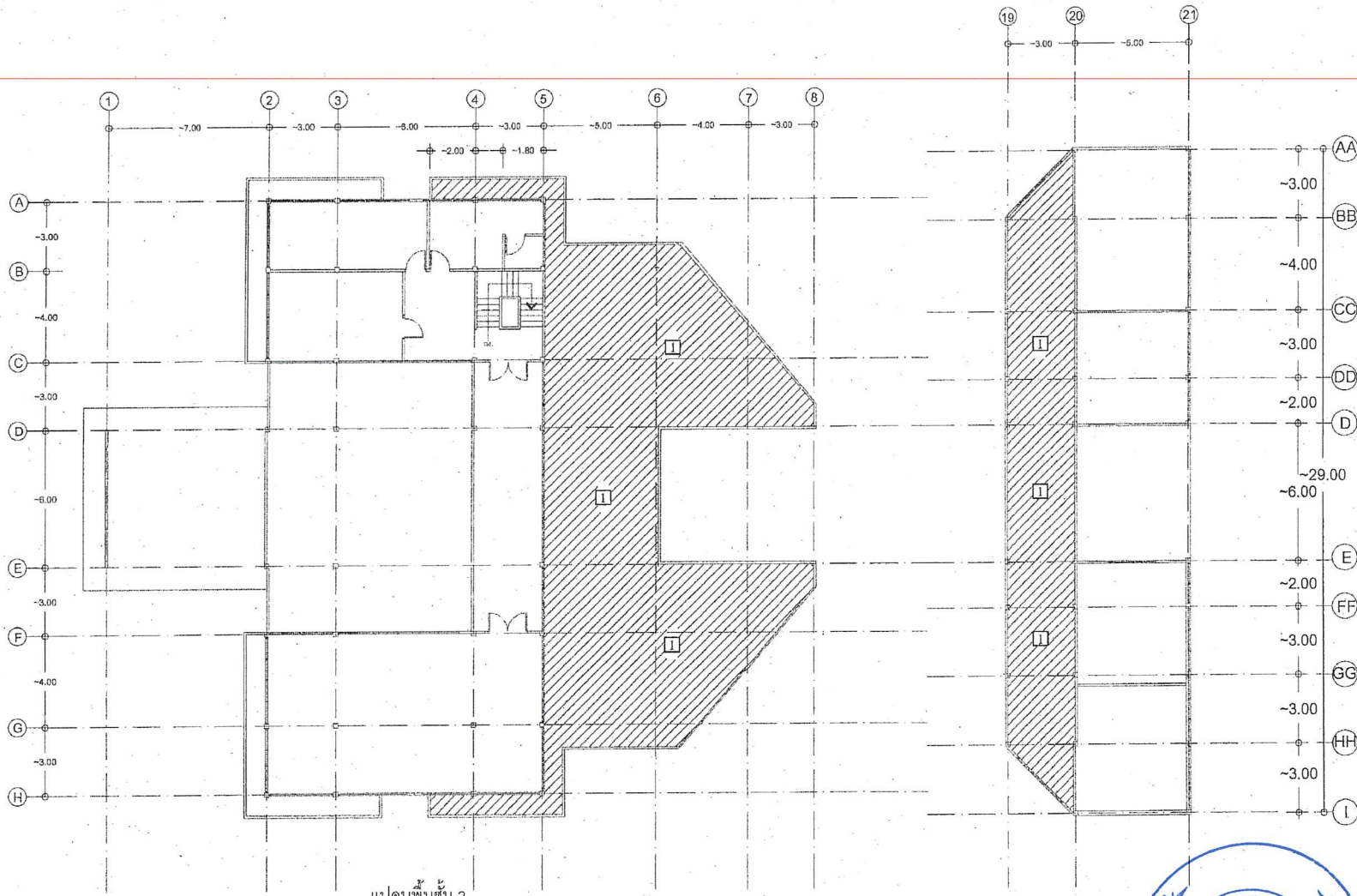
แปลนพื้นที่ 2 มาตราส่วน 1:200
