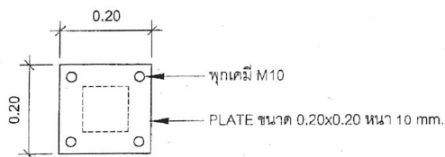
แบบขยาย PLATE 1
