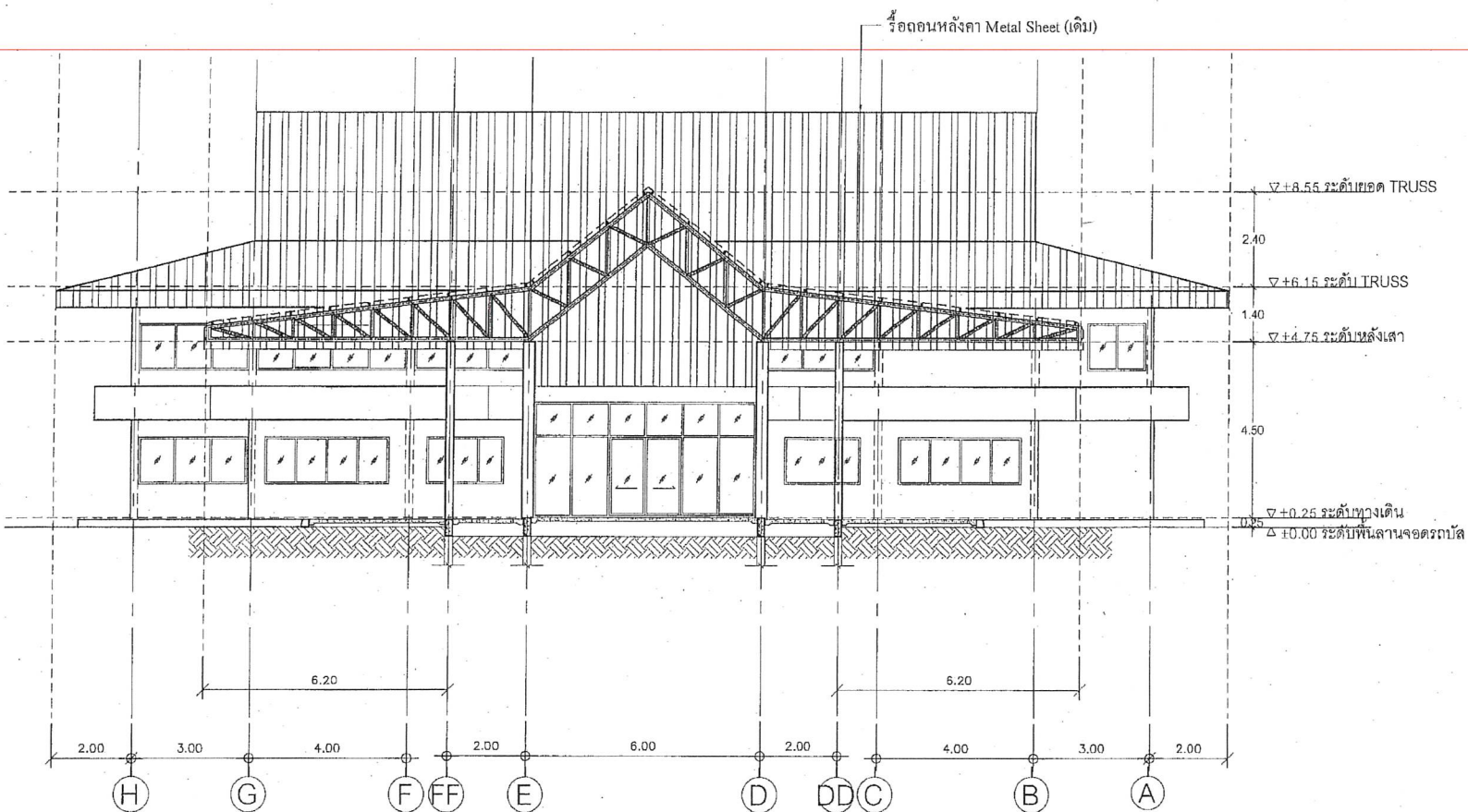
รูปตัด B SCALE 1 : 125
