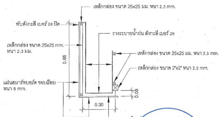
แบบขยายรางน้ำฝน
