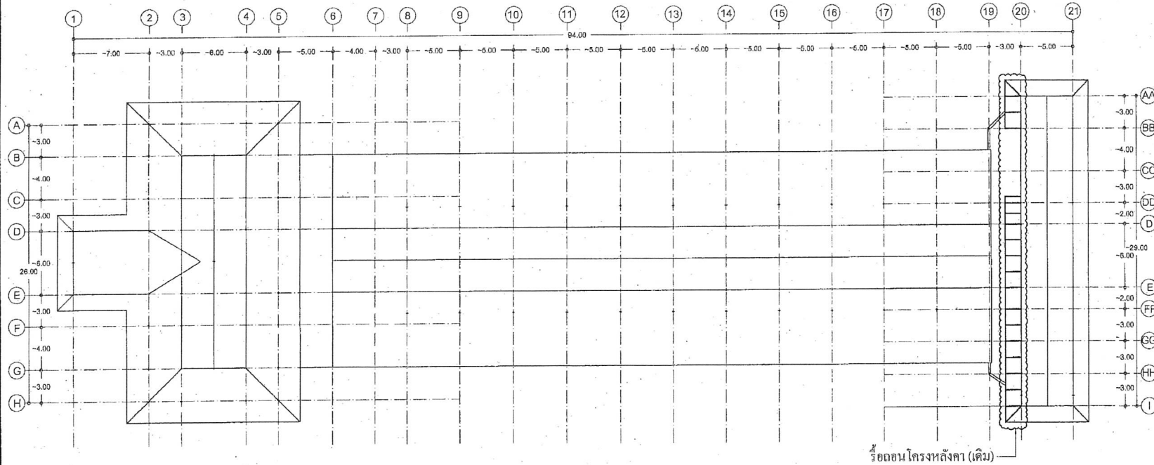
แปลนโครงหลังคาเดิม มาตราส่วน 1: 350
