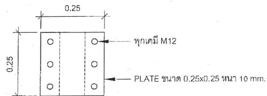
แบบขยาย PLATE 2
